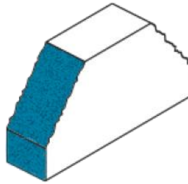
Зеленый кирпич Трапеция (1) 210x120x65 мм. 336 шт. в поддоне
