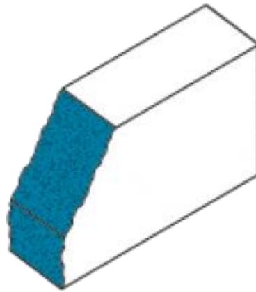
Черный кирпич Фигурный (2) 230x120x65 мм. 336 шт. в поддоне
